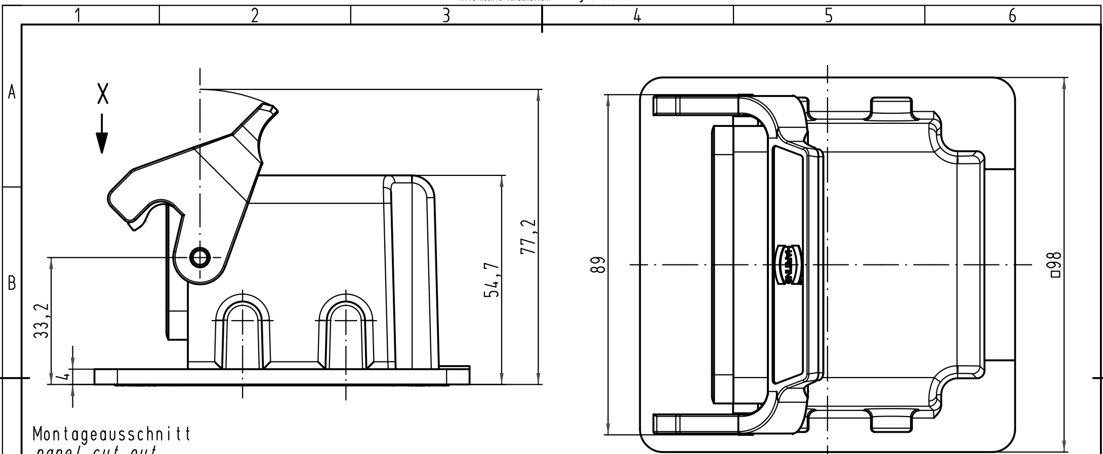
Gehäuse ohne Oberfläche housing without coating
